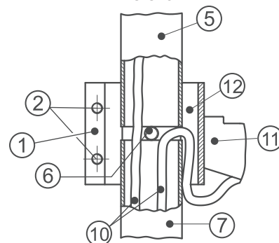
Ansicht Z
